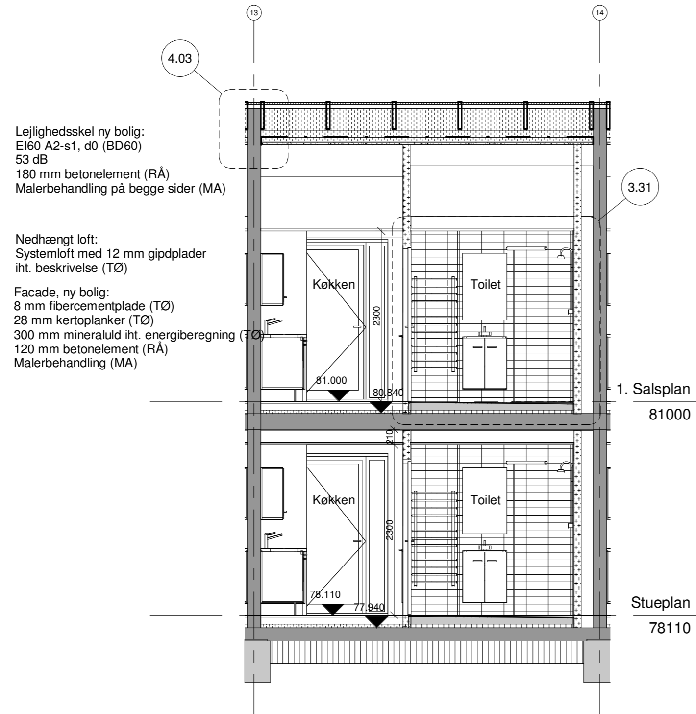
Længdesnit B-B (ny boligbygning)
